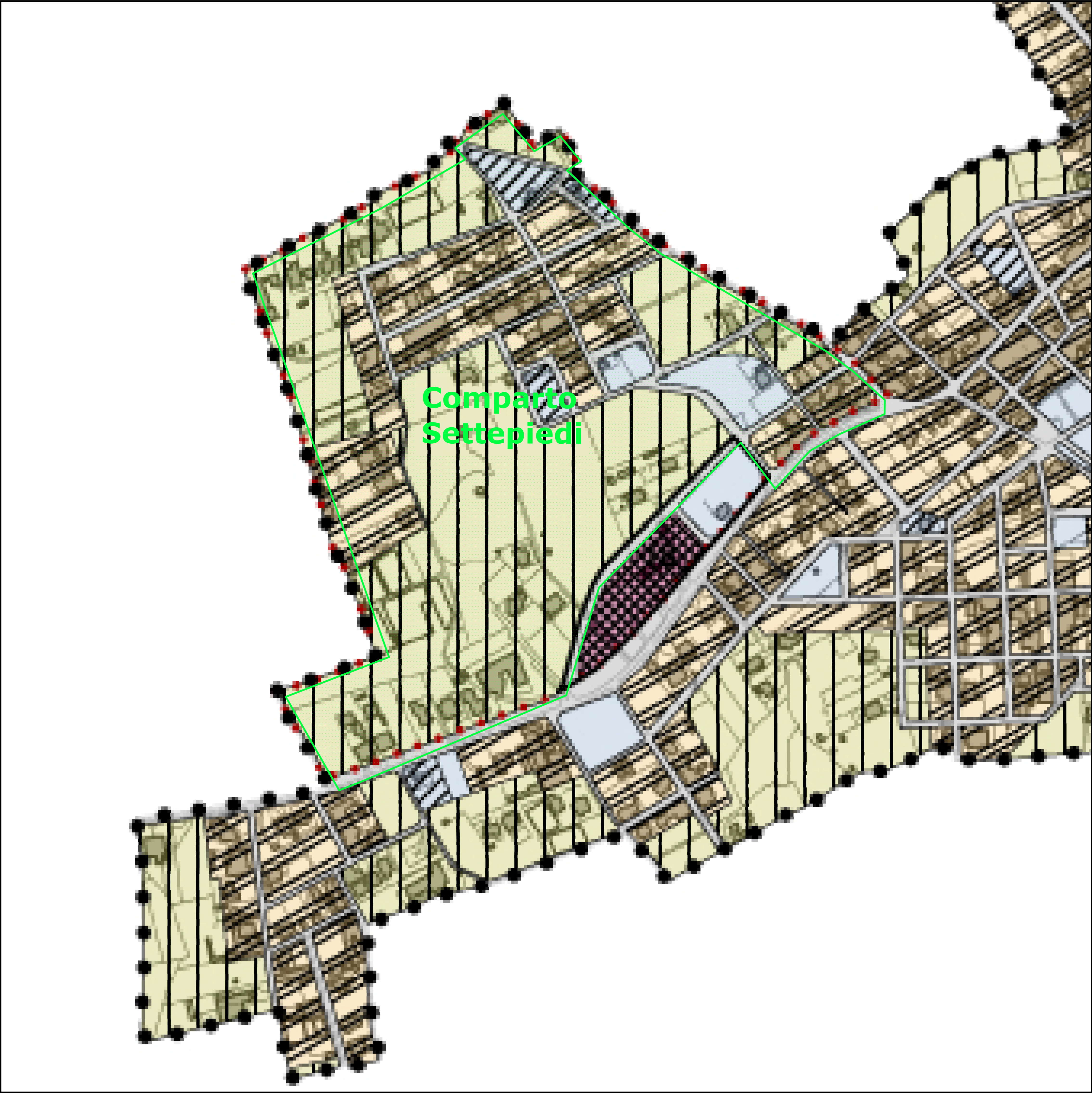
Sovrapposizione Comparto Settepedi su P.R.G. scala 1:1000
